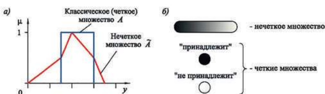
Рис. 5. Графики функций принадлежности классического (чёткого) и нечёткого множества (а) и их смысловое различие (б)
