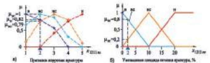
Рис. 6. Примеры графиков функций принадлежности термов переменных X_{1211ms} (а) и X_{1212ms} (б) с отображением степеней принадлежности к термам
