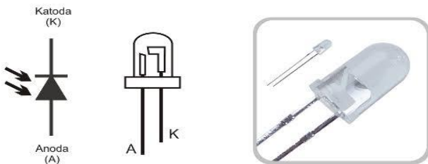
Gambar 4. Simbol dan bentuk fisik dari photodioda
