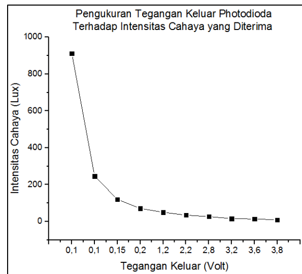
Gambar 12. Grafik hubungan tegangan keluar sensor photodiode dengan intensitas cahaya
