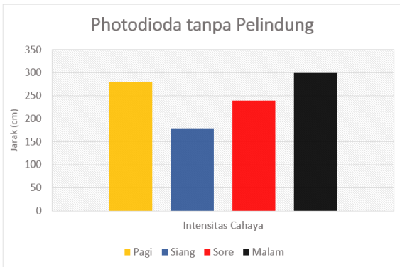
Gambar 11. Grafik deteksi api oleh sensor photodiode tanpa pelindung
