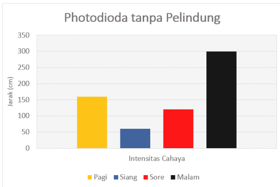
Gambar 10. Grafik deteksi api oleh sensor photodiode tanpa pelindung
