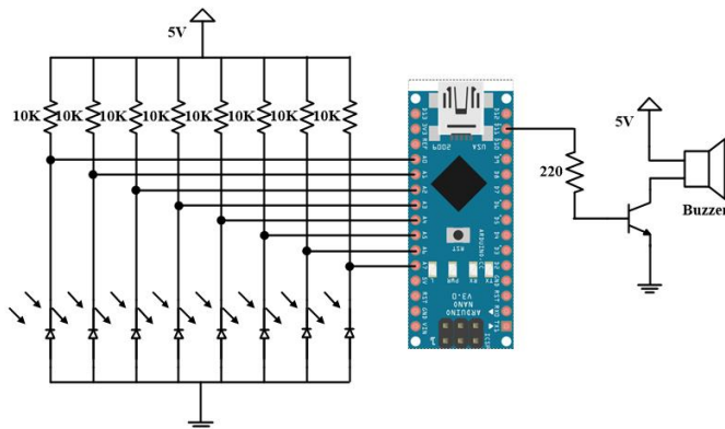
Gambar 5. Skema rangkaian sensor api menggunakan photodioda
