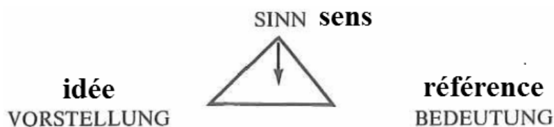
Fig. 24 – Le triangle de Frege.
