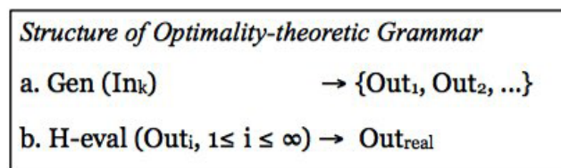
Figura 1. Processamento gramatical na TO
