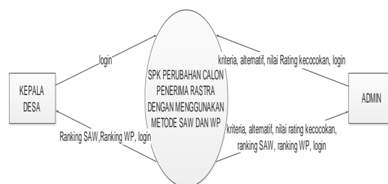
Gambar 1. Diagram Konteks
