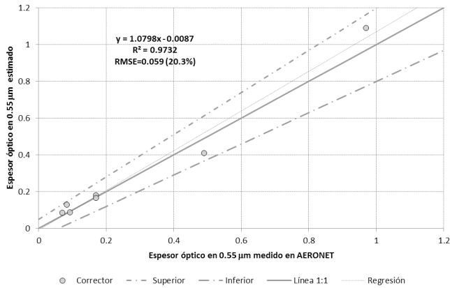
Figura 8. Comparación entre el espesor óptico en 0.55 μm medido por AERONET y el estimado por el algoritmo de corrección atmosférica, con los límites del intervalo de confianza.
