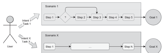
Fig. 4. User scenarios
