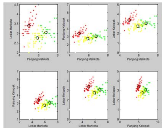
Gambar 4.2 Pengklasteran Iris Menggunakan Fuzzy C-means
