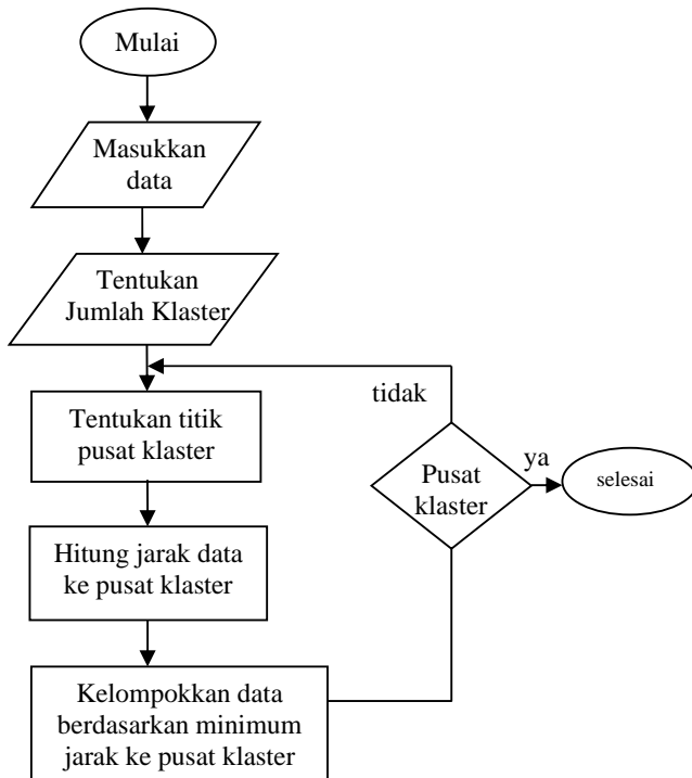
Gambar 3.1 Algoritma K-Means
