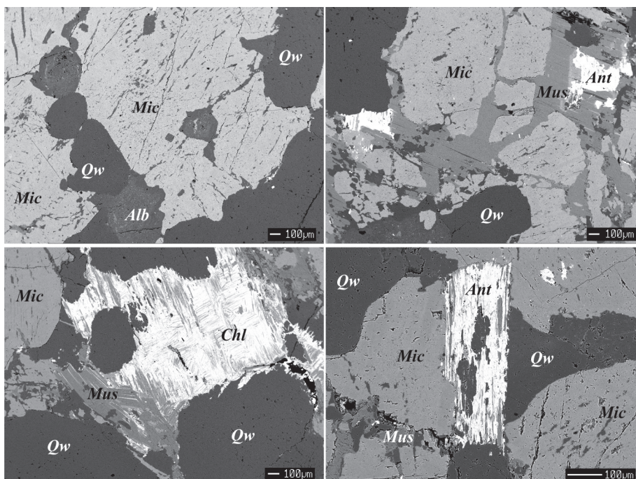
Рис. 5. Электронно-микроскопическое изображение (BSE) гранита (обр. БТ-23/1).
