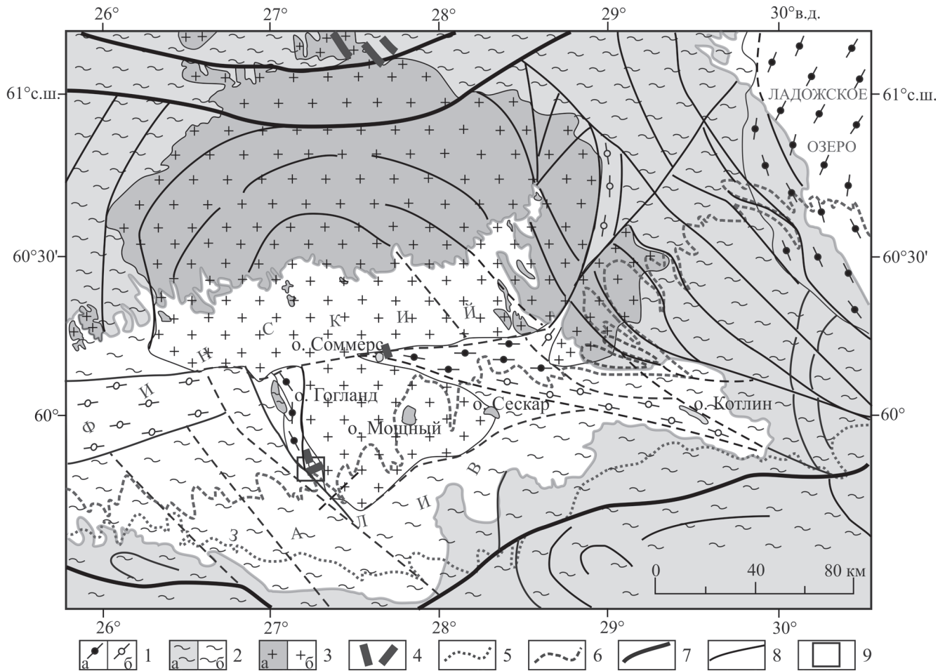
Рис. 1. Структурно-геологическое положение о. Большой Тютерс.
