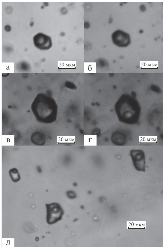
Рис. 7. Флюидные включения разных типов в кварце кварцитов о. Б. Тютерс.
