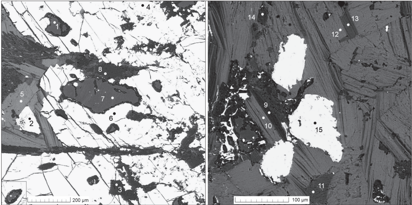
Рис. 6. Электронно-микроскопические изображения (BSE) железо-глиноземистого метасоматита (обр. БТ-8/2). 1, 7 – кварц; 2, 15 – Ti-магнетит; 4, 6 – гематит; 3, 8, 9, 14 – каолинит; 5, 10, 12 – мусковит; 11, 13 – парагонит.
