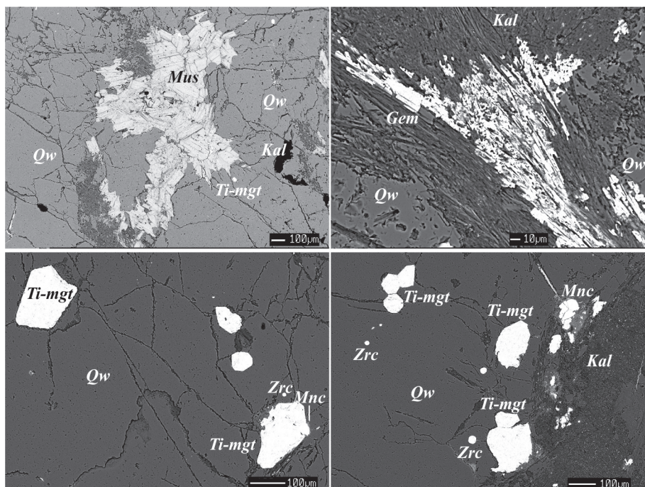
Рис. 4. Электронно-микроскопическое изображение (BSE) кварцита (обр. БТ-2/1). JEOL-8200 (ИГЕМ РАН). Kal – каолинит, Mus – мусковит, Qw – кварц, Mon – монацит, Zrc – циркон, Gem – гематит, Ti-Mgt – титаномагнетит.
