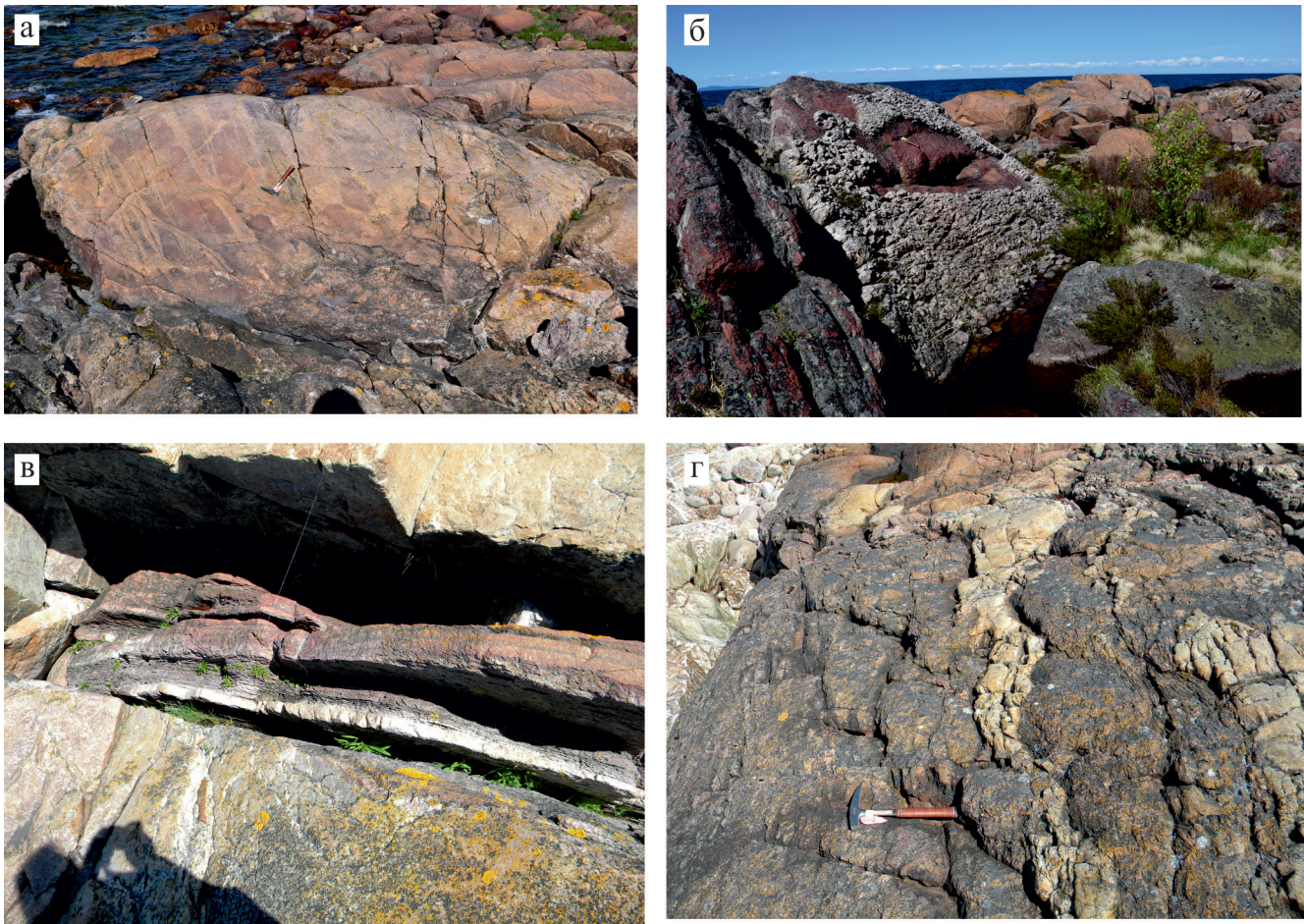
Рис. 3. Фотографии обнажений характерных разностей горных пород на о. Б. Тютерс.
