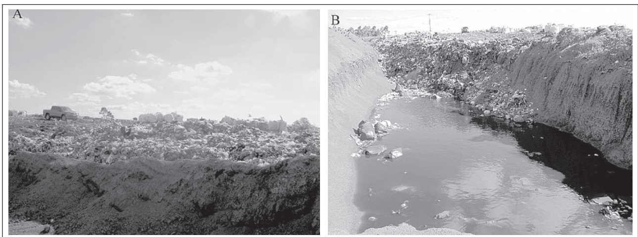
Figura 2 Resíduos à serem empurrados para a vala (A) e vala recém-aberta retendo água da chuva sobre o maciço rochoso (B) no aterro de resíduos sólidos em Pirapozinho, SP.
