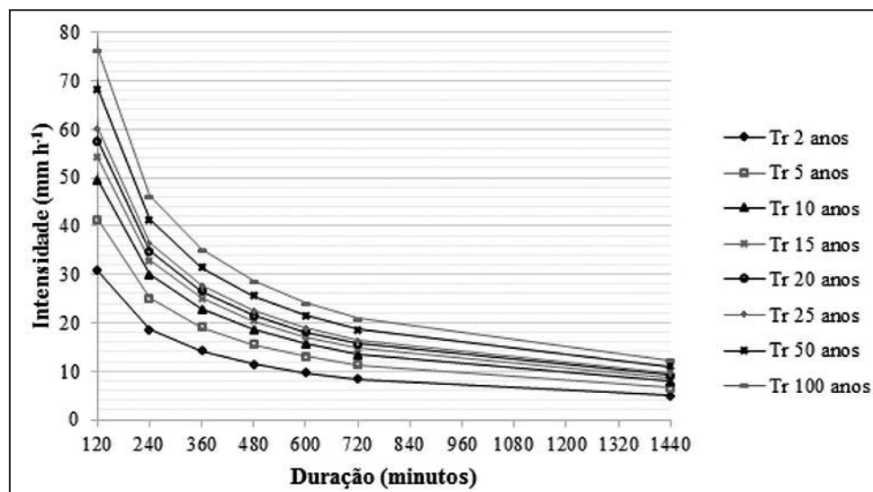
Figura 2 Curvas IDF para o município de Iraí, RS, considerando as durações de 120, 240, 360, 480, 600, 720 e 1.440 minutos e os tempos de retorno de 2, 5, 10, 15, 20, 25, 50 e 100 anos.
