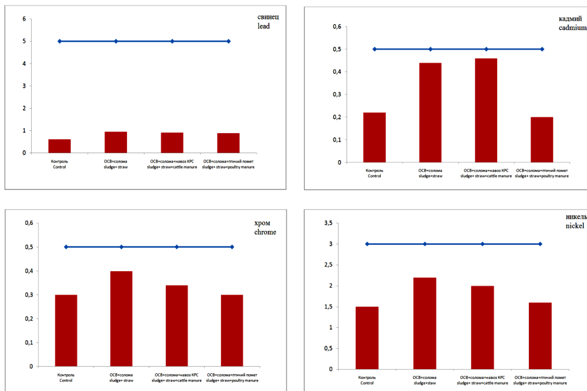
Рис.2. Динамика содержания тяжелых металлов в растениях овса при использовании видов компостов (сухая масса), мг/кг Fig.2. Dynamics of heavy metals in oat plants when using compost types (dry weight), mg/kg
