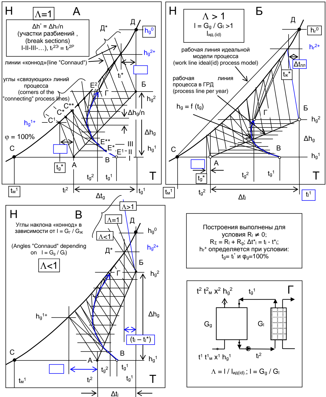
Рис. 2. Построение линии изменения состояния воздушного потока на Н-Т диаграмме влажного воздуха по высоте испарительного водоохладителя ГРД 1 при различных значениях характеристического числа \Lambda (соотношения потоков газа и жидкости l = G_{\Gamma} / G_{ж} ) и противоточной схеме контактирования потоков, при условии: R_{ж} \neq 0 [12]
