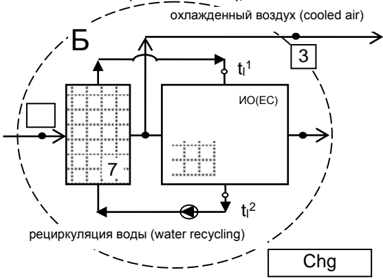
Рис. 5. Анализ работы СКВ (по рис. 1) на основе воздухоохладителя Chg при различных начальных влажностях воздуха x_r^1 (при l = 1,0 ) 1
