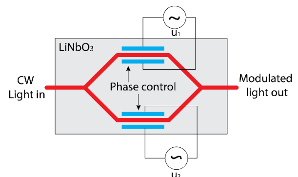
Fig. 3. Mach-Zehnder modulator
