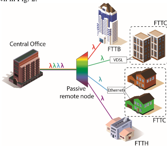
Fig. 2. Structure of WDM-PON
