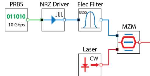
Fig. 6. IMDD transmitter
