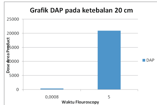
Gambar 4 DAP pada ketebalan phantom 20 cm
