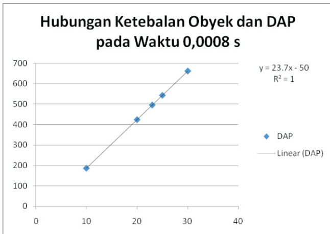
Gambar 7 Grafik DAP pada waktu 0,008 menit
