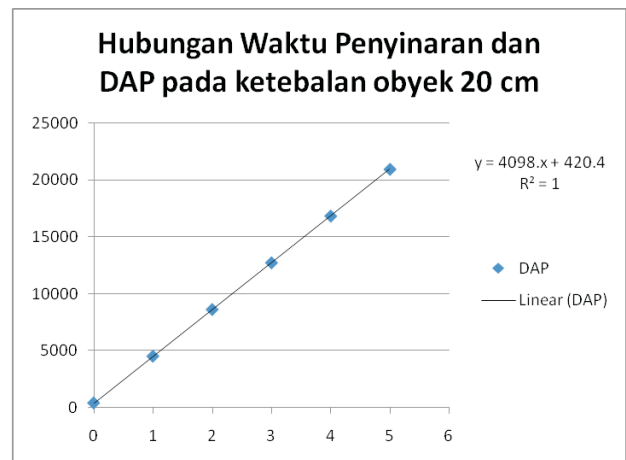
Gambar 6 Grafik DAP pada ketebalan phantom 20 cm
