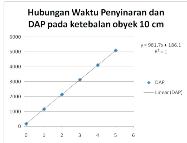
Gambar 5 Grafik DAP pada ketebalan phantom 10 cm
