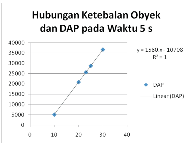
Gambar 8 Grafik DAP pada waktu penyinaran 5 menit
