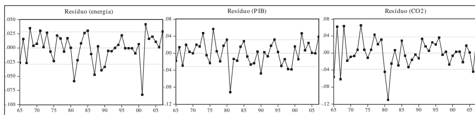
Figura 3: Resíduos do modelo VECM
