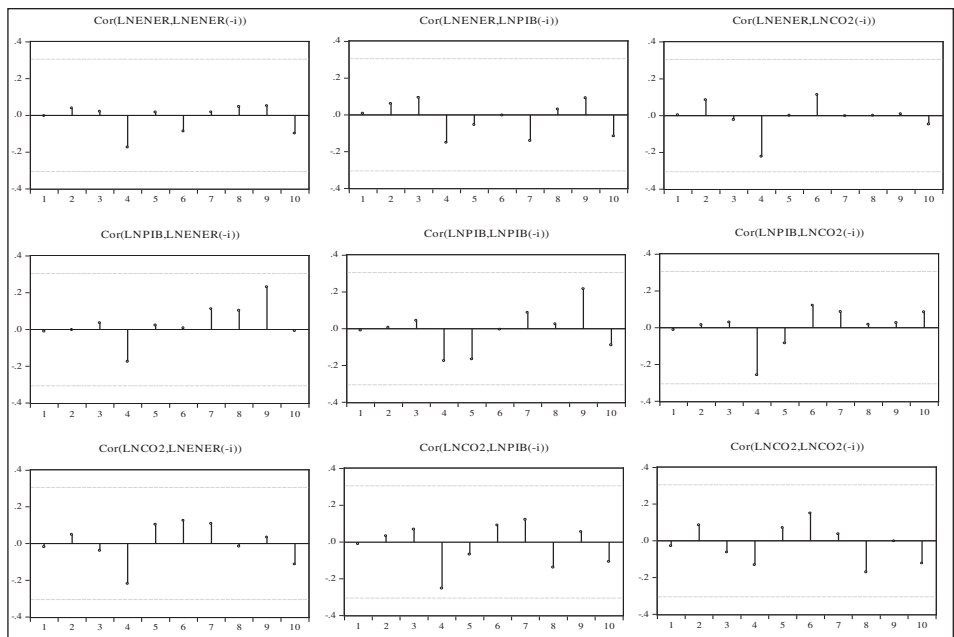
Figura 4: Correlograma dos resíduos do VECM
