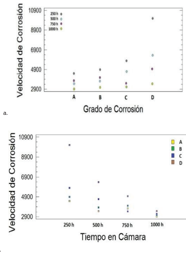
Gráfico 3. a. Comportamiento de la variable velocidad de corrosión en función del grado de corrosión y b. Comportamiento de la variable velocidad de corrosión en función del tiempo de exposición en cámara de niebla salina neutra. A: Grado de corrosión A; B: Grado de corrosión B; C: Grado de corrosión C; D: Grado de corrosión D.
