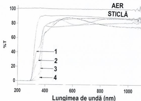
Fig.2. Dependenta spectrală a transmitanței straturilor de ZnO obținute pentru diferite volume ale soluției pulverizate. V, ml: 1 – 5; 2 – 10; 3 – 20; 4 – 40.
