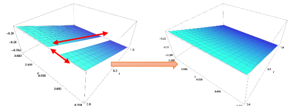
(a) ADM u(x, t) (b) ADM-Padé u(x, t)
