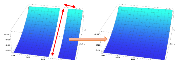
(a) ADM v(x, t) (b) ADM-Padé v(x, t)
