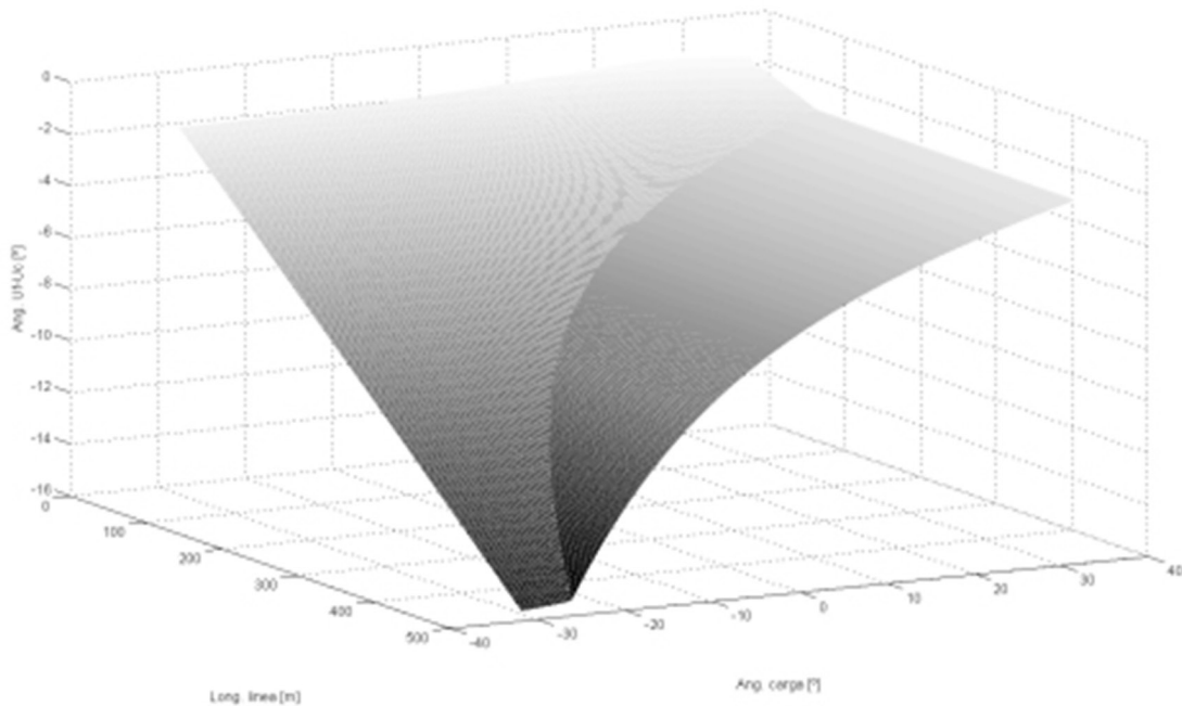
FIG. 2: ÁNGULO ENTRE LOS FASORES V_f Y V_c , EN FUNCIÓN DEL ÁNGULO DE LA CARGA Y LA LONGITUD DE LA LÍNEA.
