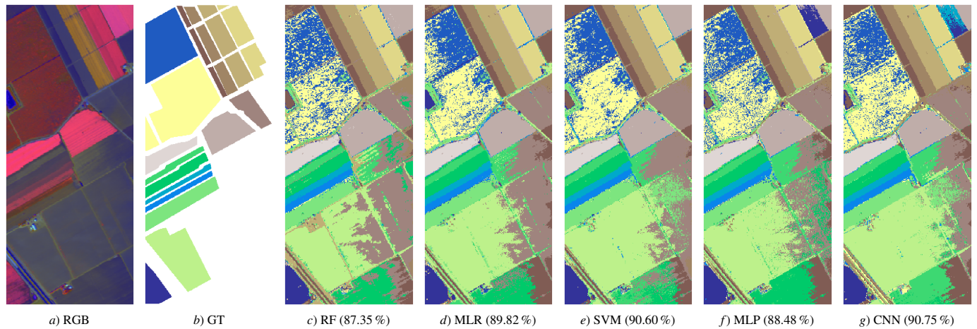
Figura 3: Mapas de clasificación para el dataset hiperespectral Salinas Valley (SV). El primer mapa (a) representa una imagen sintética en RGB. El segundo (b) contiene la verdad terreno de los datos. Finalmente, el resto de las imágenes (c) a (g) muestran los mapas de clasificación correspondientes a la Tabla3. El porcentaje de acierto ó Overall Accuracy (OA) se muestra entre paréntesis.
