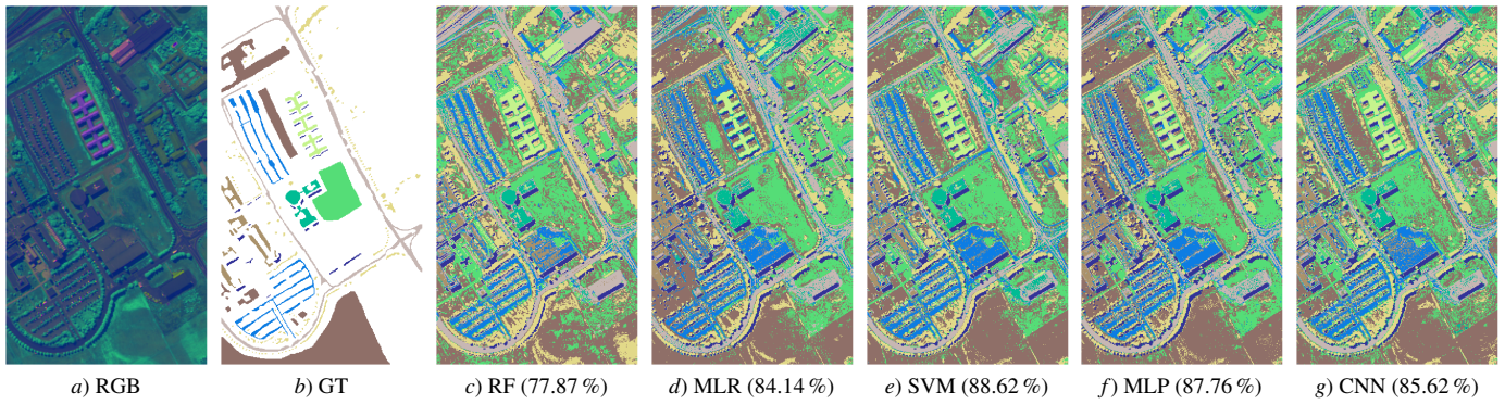
Figura 2: Mapas de clasificación para el dataset hiperespectral Pavia University (PU). El primer mapa (a) representa una imagen sintética en RGB. El segundo (b) contiene la verdad terreno de los datos. Finalmente, el resto de las imágenes (c) a (g) muestran los mapas de clasificación correspondientes a la Tabla3. El porcentaje de acierto ó Overall Accuracy (OA) se muestra entre paréntesis
