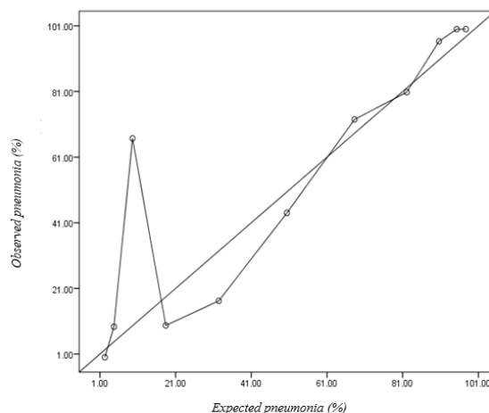
Gambar 1. Plot kalibrasi skor A 2 DS 2
