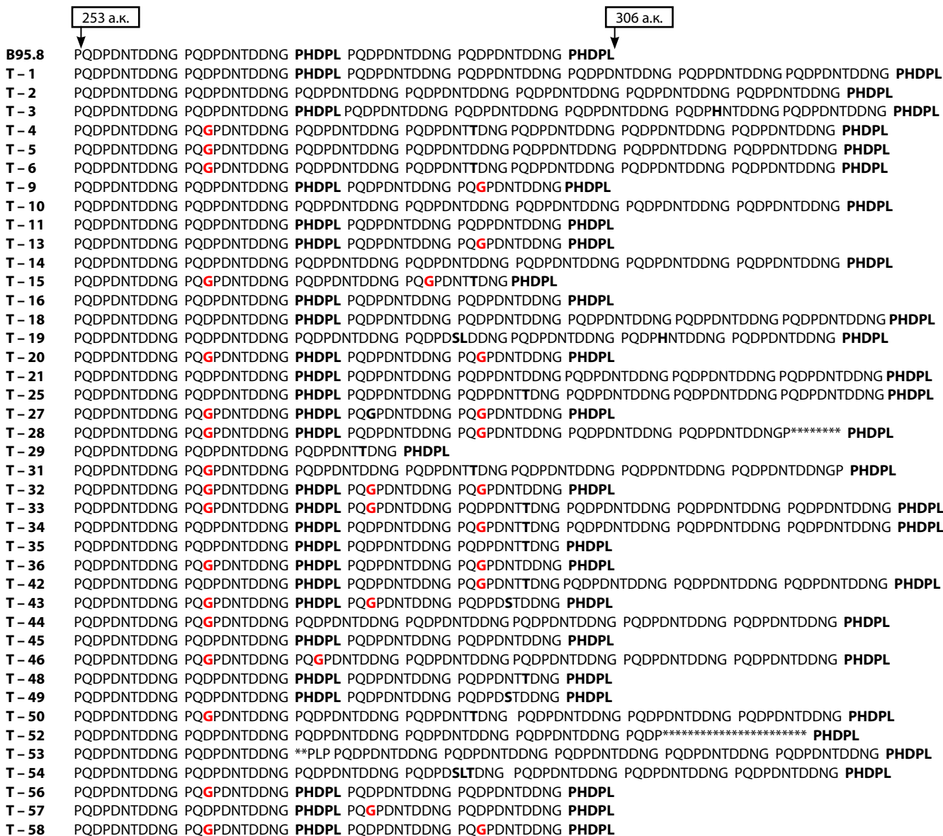
Рис. 1. Варианты 11 а.к. повторов С-терминального домена в изолятах LMP1 у представителей этнических татар г. Казани. T1...T58 – кодовое обозначение изолятов LMP1; QQDPDNTDDNG – повторяющиеся элементы 11 а.к.; PHDPL – вставка 5 а.к. последовательностей; D→G – точечные мутации в области 11 а.к.
