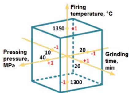
Fig. 1 The arrangement of experiments of type 2 3 in three-dimensional space 1. ábra 23 háromfaktoros teljes faktoriális kísérleti tervelrendezés három dimenziós térben ábrázolva
