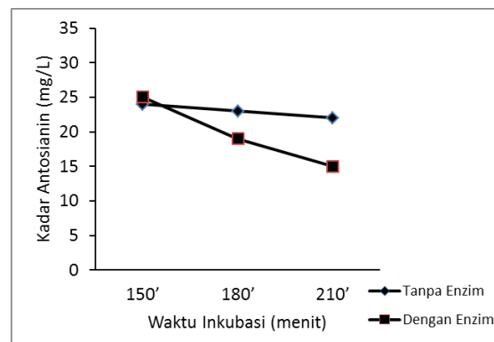
Gambar 4. Grafik kadar antosianin dengan dan tanpa enzim AbfA dengan waktu inkubasi bervariasi pada Suhu 70°C
