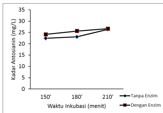
Gambar 3. Grafik kadar antosianin dengan dan tanpa enzim AbfA dengan waktu inkubasi bervariasi pada Suhu 60°C.
