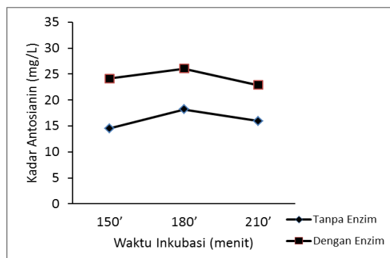
Gambar 1. Grafik kadar antosianin dengan dan tanpa enzim AbfA dengan waktu inkubasi bervariasi pada Suhu 40°C.
