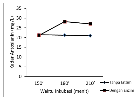
Gambar 2. Grafik kadar antosianin dengan dan tanpa enzim AbfA dengan waktu inkubasi bervariasi pada Suhu 50°C.
