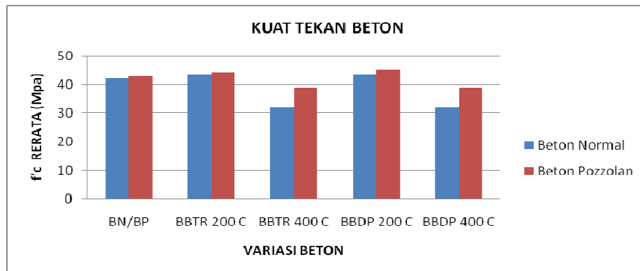
Gambar 2 Grafik kuat tekan beton
