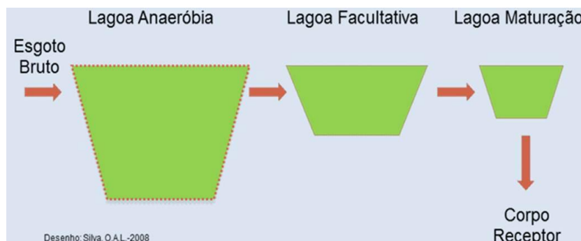
Figura 02. Esquema simplificado de uma estação de tratamento de esgoto do tipo secundário. Fonte: CAERN, 2017.
