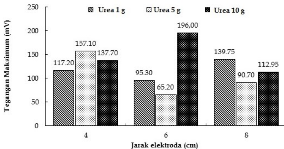
Gambar 3. Tegangan listrik maksimum yang dihasilkan masing-masing perlakuan
