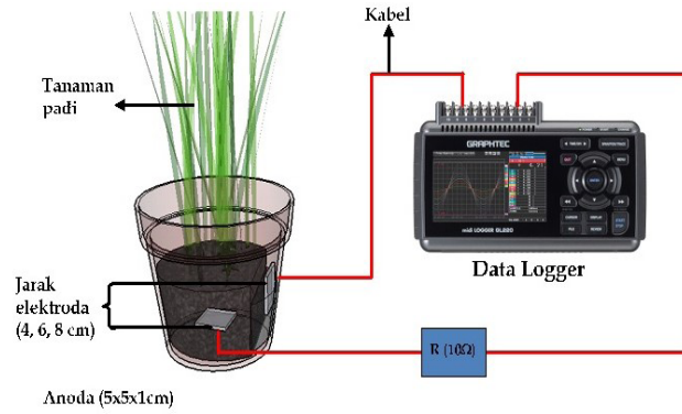
Gambar 1. Skema rangkaian PMFC padi
