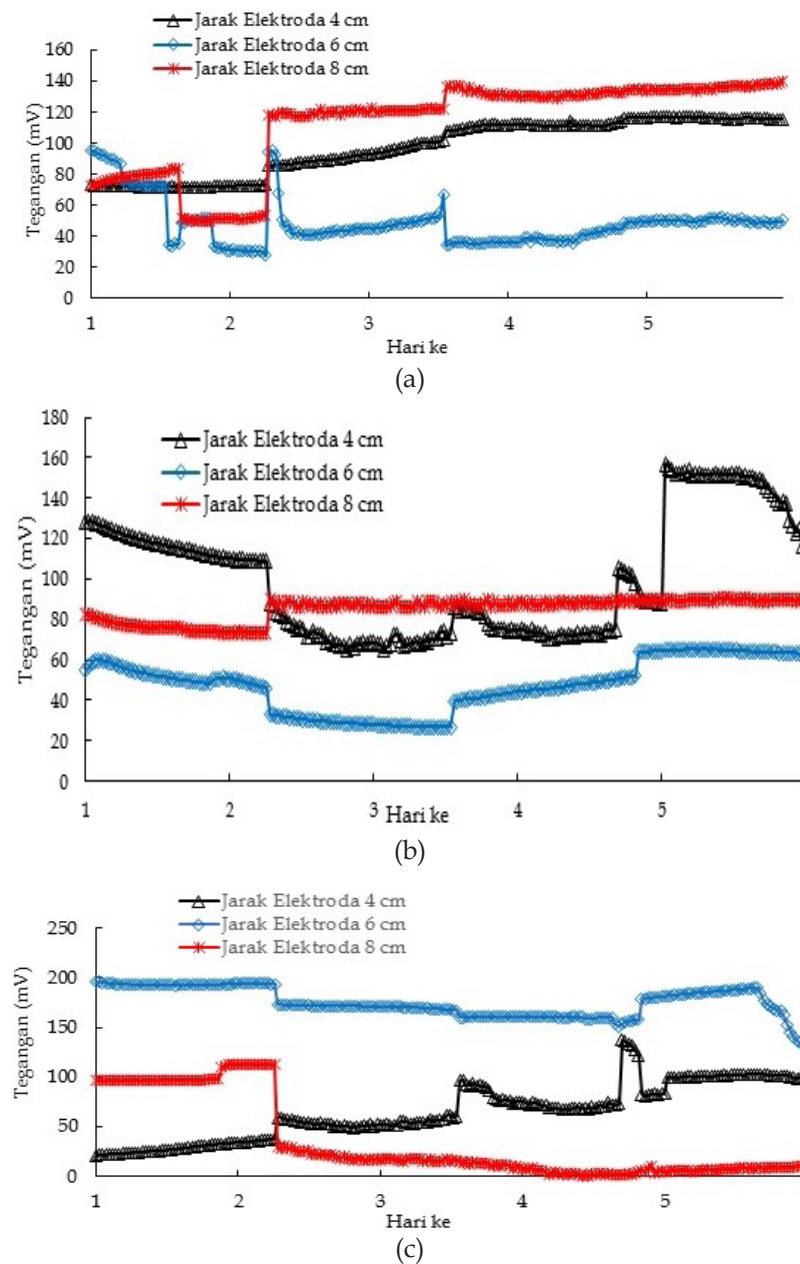
Gambar 2. Tegangan listrik yang dihasilkan pada variasi perlakuan jarak elektroda selama 5 hari. (a) 1 g urea; (b) 5 g urea; dan (c) 10 g urea
