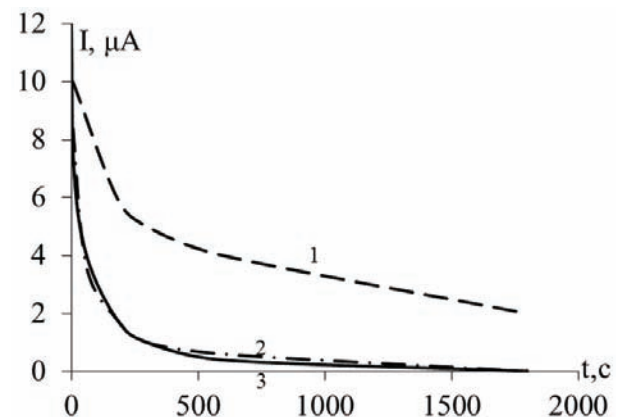
Рис. 3. Падение коррозионного тока в биметаллическом имплантате на основе титана в сочетании с платиной (1), серебром (2) и золотом (3).
