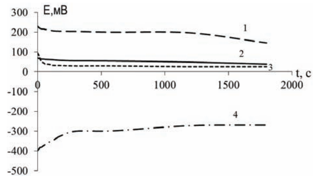
Рис. 2. Изменения во времени величин потенциалов на платиновом (1), серебряном (2), золотом (3) и титановом (4) электродах – составных частях имплантатов, измеренные в фосфатно-щелочном буферном растворе (pH 7,4) относительно хлорсеребряного электрода сравнения.
