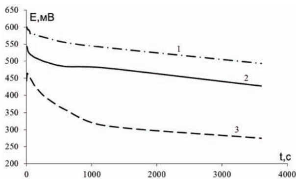
Рис. 1. Падение потенциалов платинового (1), золотого (2) и серебряного (3) электродов, измеренных относительно основного (титанового) электрода в фосфатно-щелочном буферном растворе, pH 7.4.
