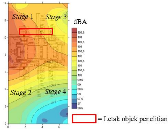
Gambar 1. Noise mapping pada area kompresor
