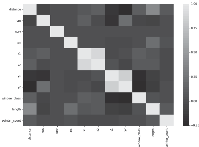
Fig. 5. Gestures parameters correlation
