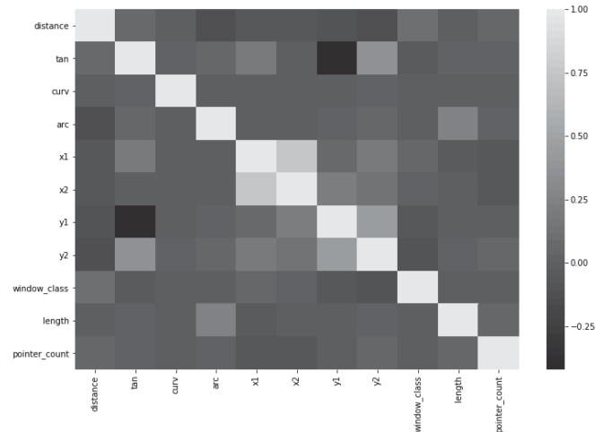
Fig. 7. Motion gestures parameters correlation
