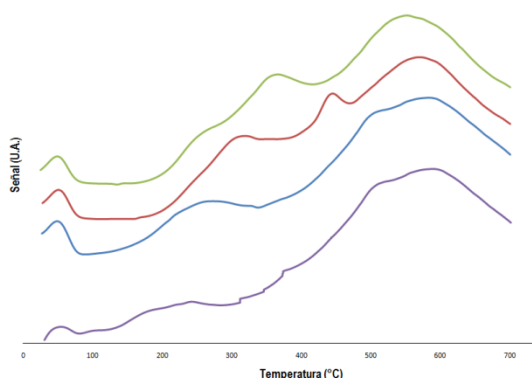
Figura 1: curvas de TPR para el catalizador Pt/C, PtBi 0.25 /C, PtBi 0.50 /C y PtBi 1.00 /C.
