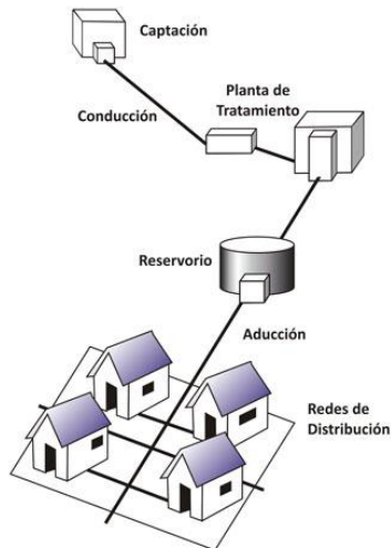
Figura 1: Sistema de abastecimiento por gravedad con tratamiento.
