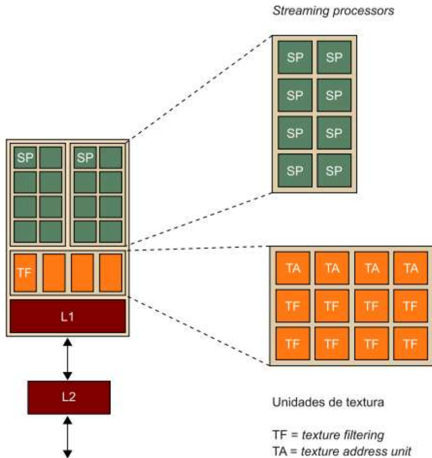
Ilustración 14 Streaming processors y unidades de textura que forman un bloque en la arquitectura G80 de Nvidia
