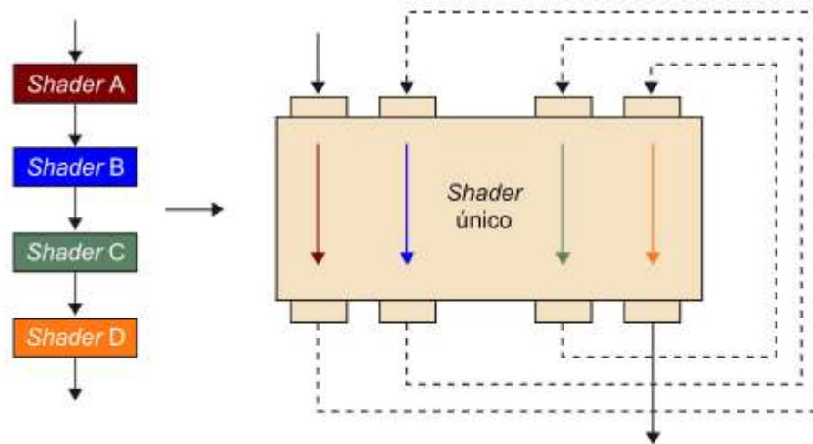
Ilustración 13 Comparación entre un pipeline secuencial y el cíclico de la arquitectura unificada
