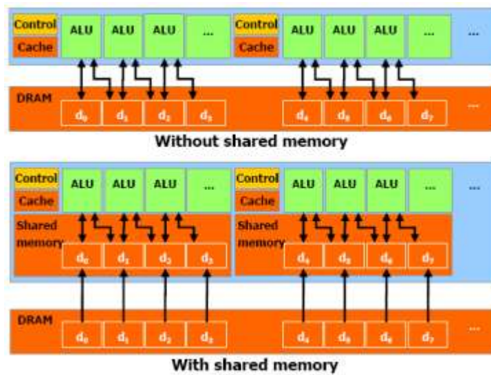
Ilustración 22 División de memoria en CUDA
