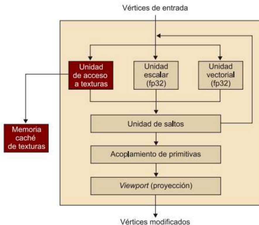
Ilustración 10 Procesador de vértices de la serie GeForce 6 de Nvidia
