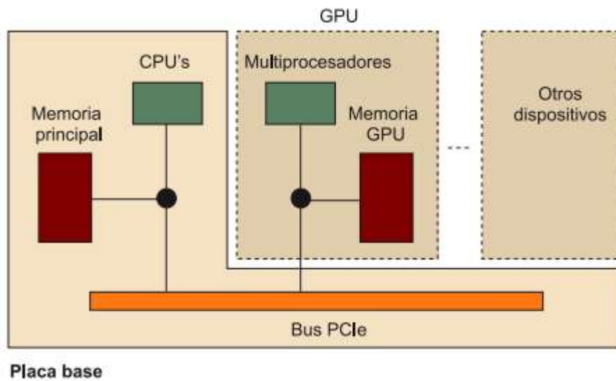
Ilustración 8 Interconexión entre CPU y GPU mediante PCIe
