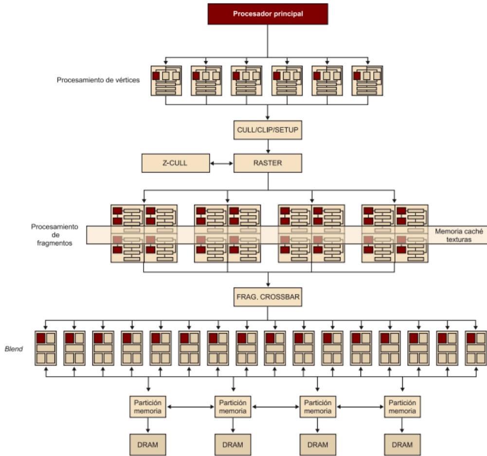
Ilustración 9 Esquema de la arquitectura de la GPU GeForce 6 de Nvidia
