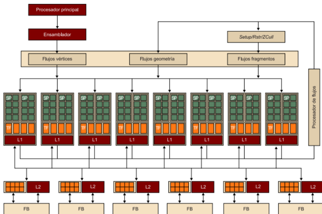
Ilustración 12 Arquitectura unificada de la serie G80 de Nvidia
