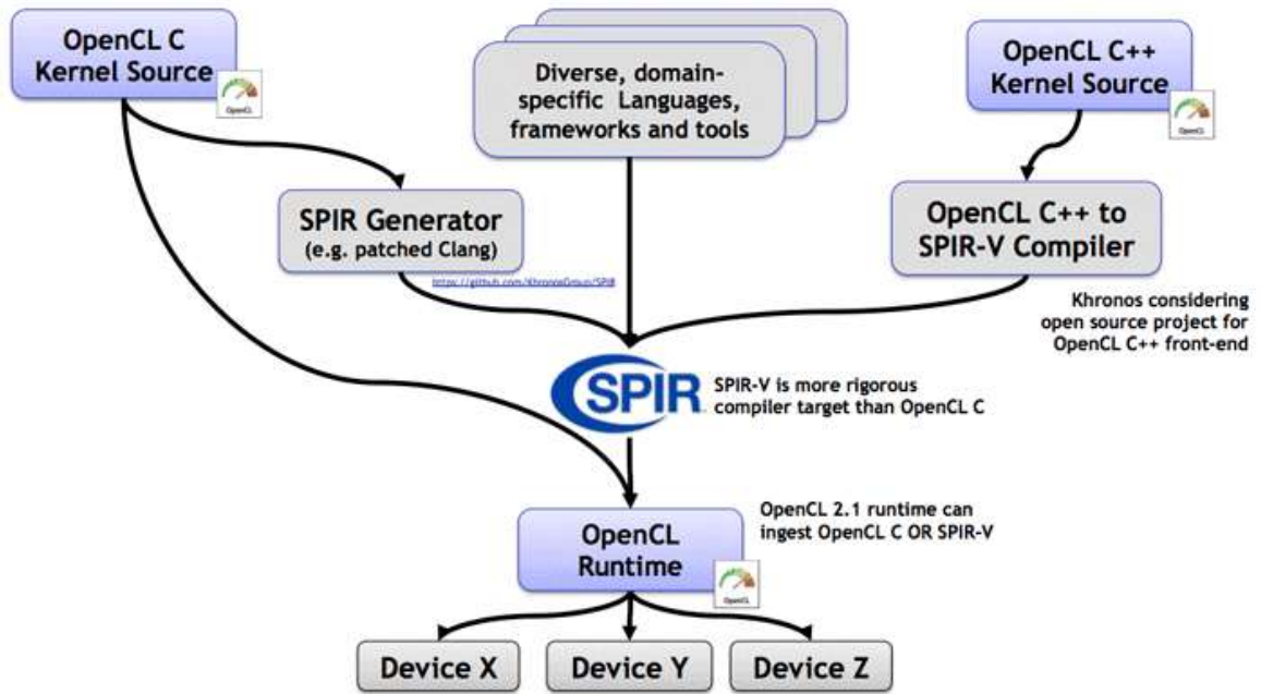
Ilustración 19 Ecosistema de Compilación de OpenCL 2.1
