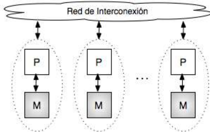
Ilustración 5: Arquitectura de una máquina con paso de mensajes
