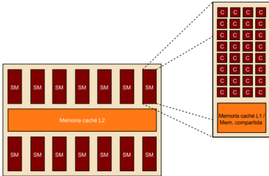
Ilustración 16 Esquema simplificado de la arquitectura Fermi
