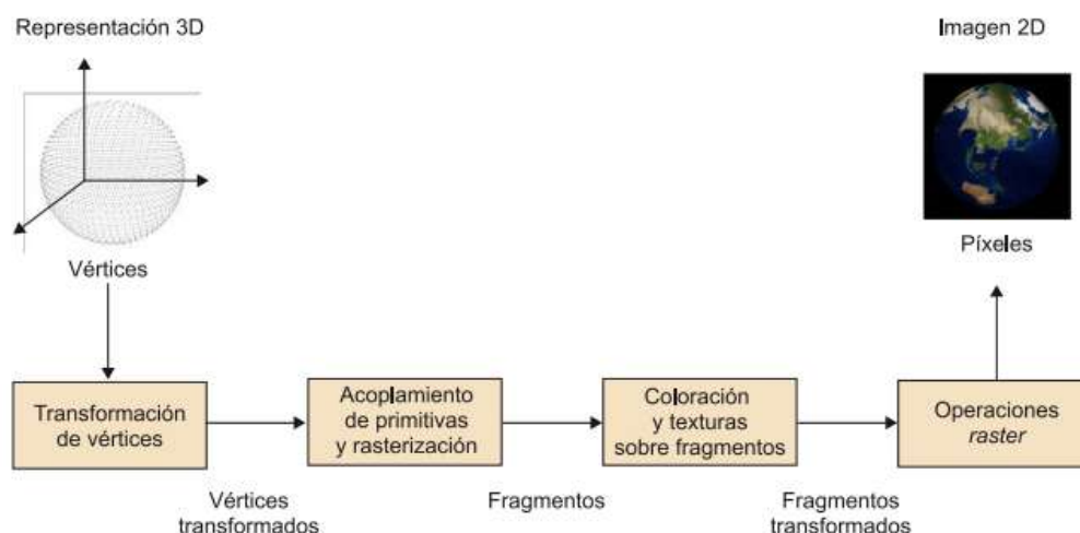
Ilustración 6 Funcionalidades del Pipeline Gráfico
