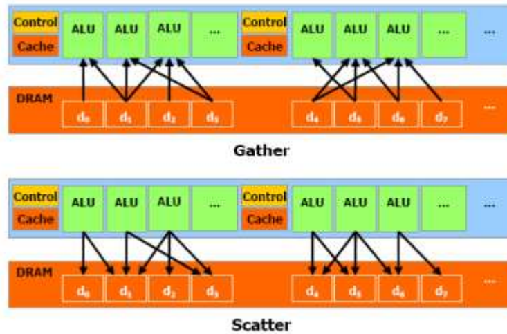
Ilustración 21 Repartición de memoria en CUDA
