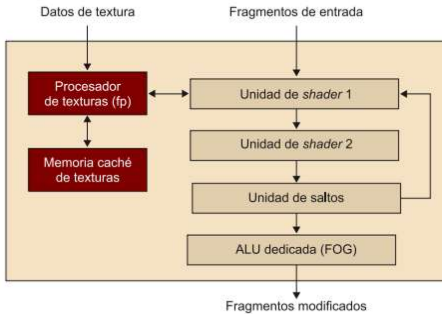
Ilustración 11 Procesador de fragmentos de la serie GeForce 6 de Nvidia
