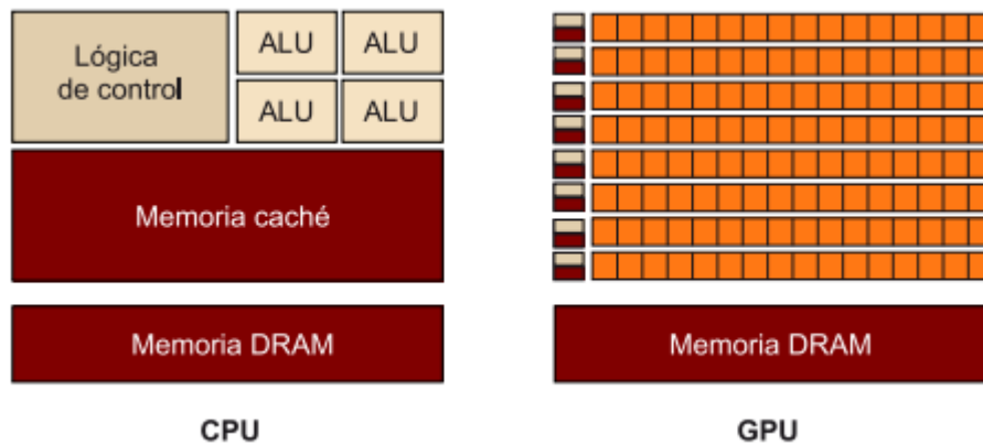
Ilustración 7 Comparativa de la superficie dedicada típicamente a computación, memoria y lógica de control para CPU y GPU
