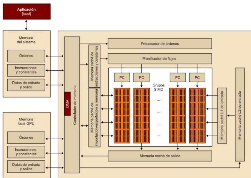
Ilustración 17 Diagrama de bloques de la arquitectura de la serie R600 de AMD
