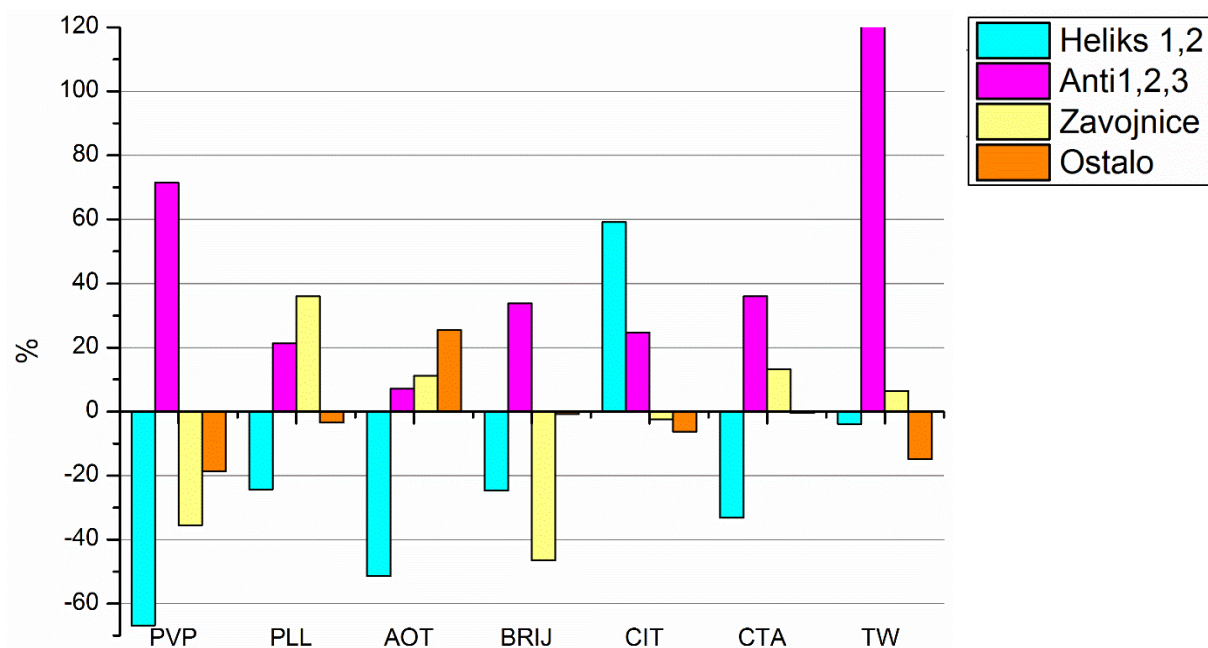
Slika 47. Promjena strukture AGP u interakciji s AgNP10 u koncentraciji od 100 µM.
