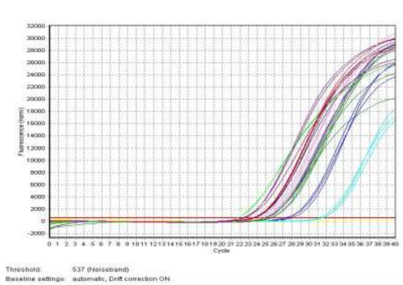
Figura 14. diagramma della fluorescenza dei cicli di amplificazione con andamento sigmoide; numero di cicli di PCR e grado di fluorescenza.
