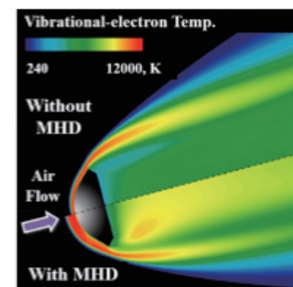
図2: MHDによる再突入時の流れの制御
