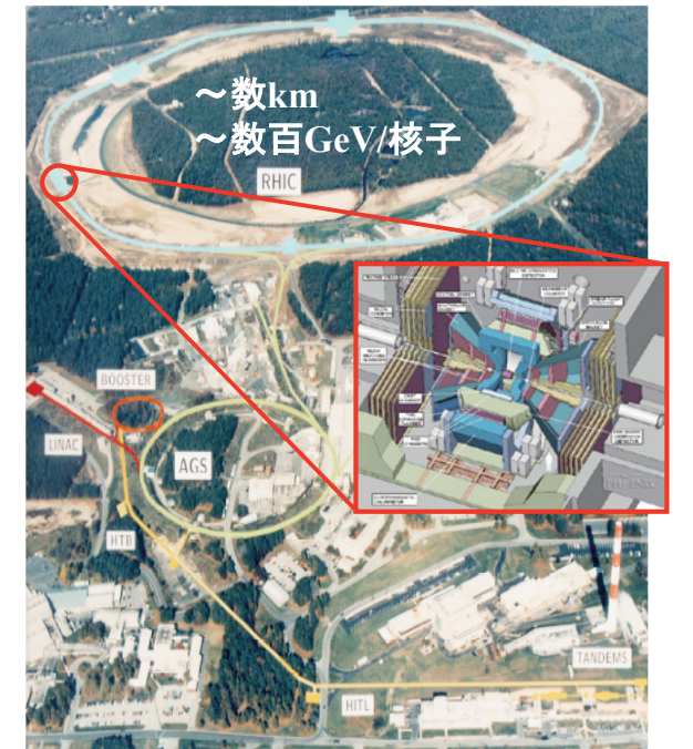
図 3 : BNL 研究所の RHIC 加速器と PHENIX 実験の検出器
