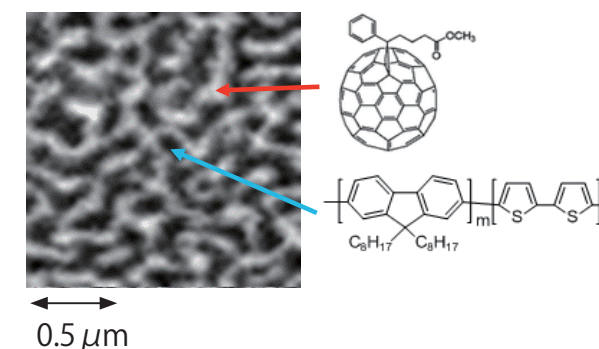
図3: 有機薄膜太陽電池の分子構造
