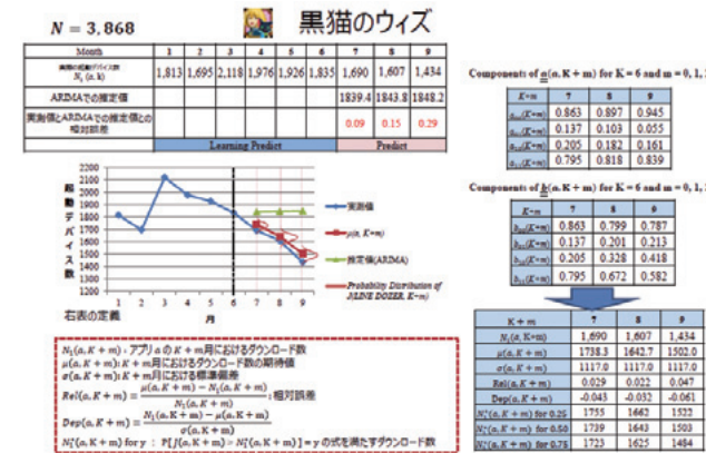
図3：開発中のアルゴリズムによるダウンロード数予測の例 ARIMA モデルよりも精度の高い予測が可能
