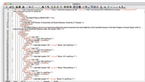
図2：上記システムから出力した TEI 形式 XML ファイル
