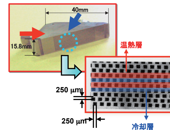
図2：手のひらサイズの熱交換器：(左上)熱交換器本体、(右下)断面図
