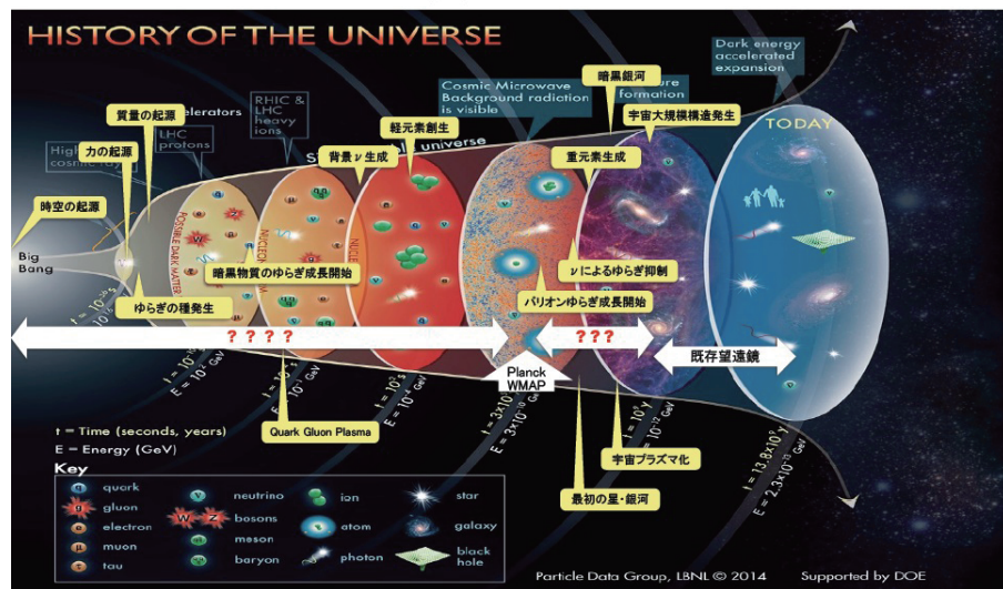
図 1: 宇宙史。横軸が時間軸、縦軸が空間軸で、ビッグバン宇宙の膨張とともに、相が変わっていくことを示す。
