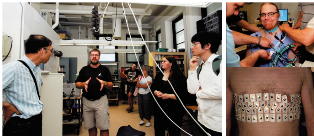
図2：ヘルシンキ大学 Samuli Siltanen 教授が自ら体表の電流測定テスト
