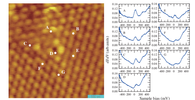
図 2: N 含有グラフェンの STM 像と STS スペクトル (STM: 走査トンネル顕微鏡、STS: 走査トンネル分光法)
