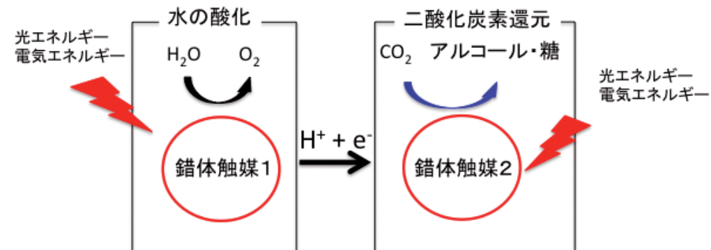
図2：錯体触媒による水の酸化と二酸化炭素の還元
