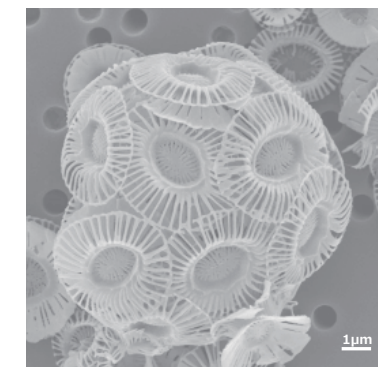
図2：円石藻類の一種。(スケールバーは1000分の1mm)
