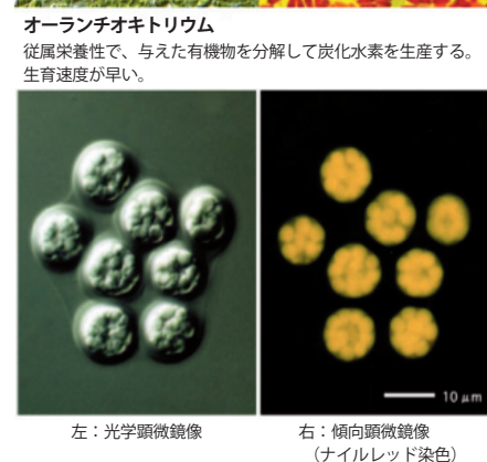
図2: 我々が着目している藻類
