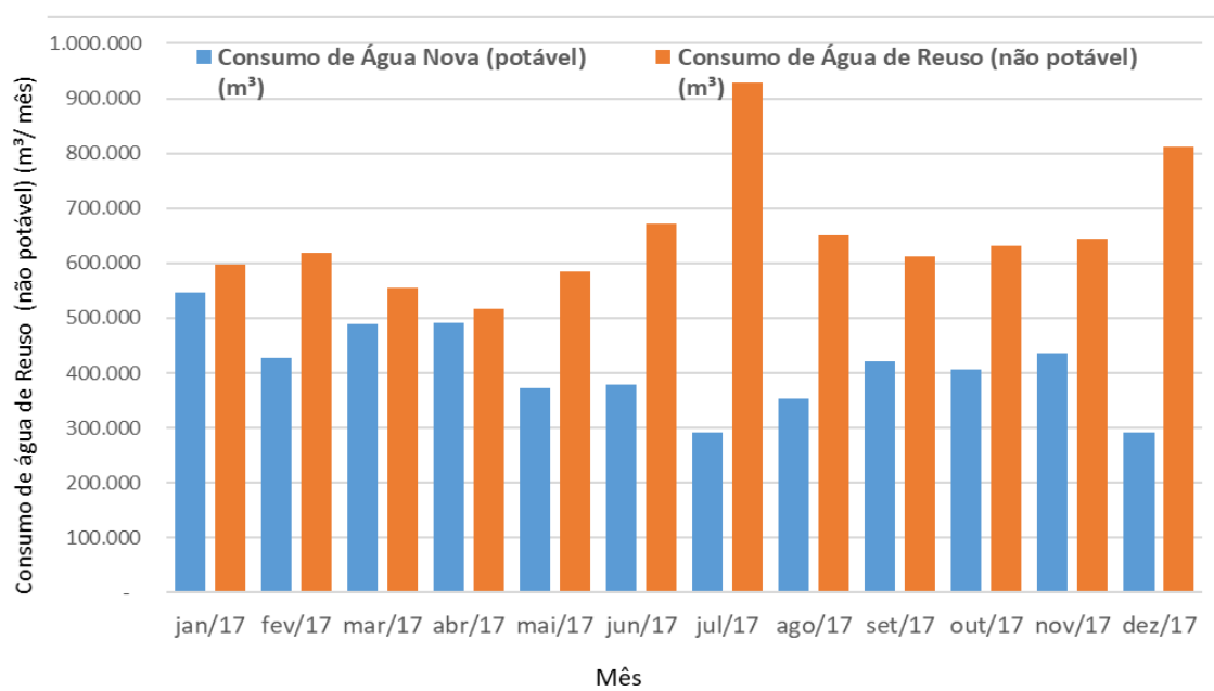
Figura 29 – Série histórica das vazões de consumo de água de Reuso (não potável) na Unidade de Tubarão em 2017
