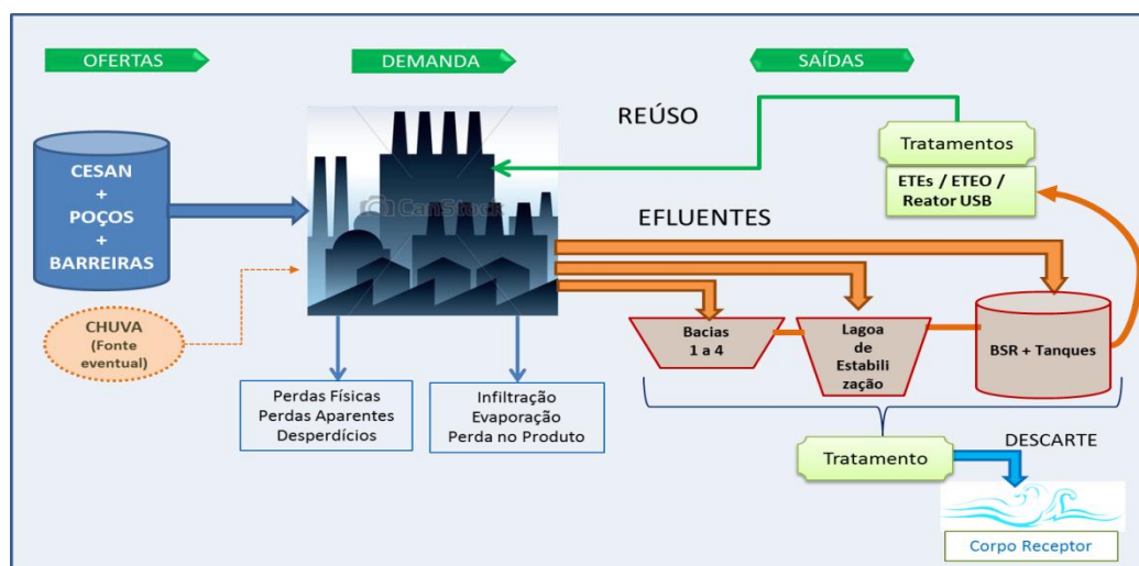
Figura 6 - Esquemático do fluxo de água simplificado da Unidade de Tubarão
