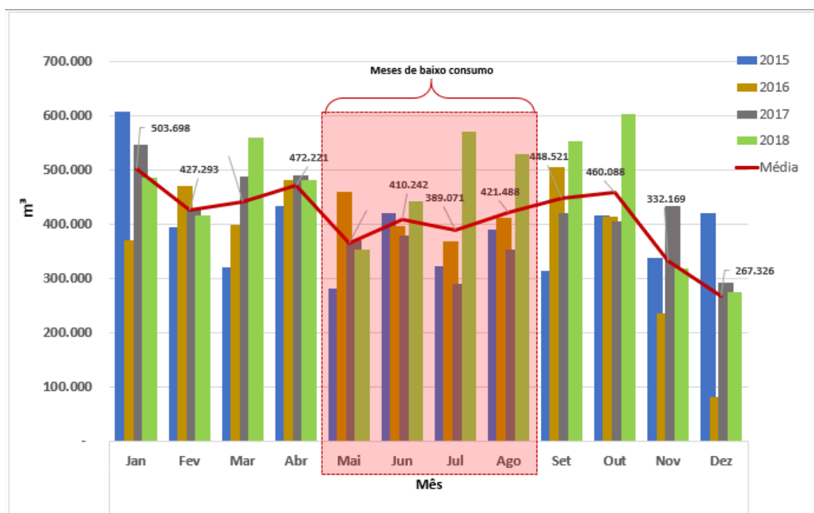
Figura 23 - Consumo mensal de Água Nova em Tubarão nos anos de 2015 a 2018
