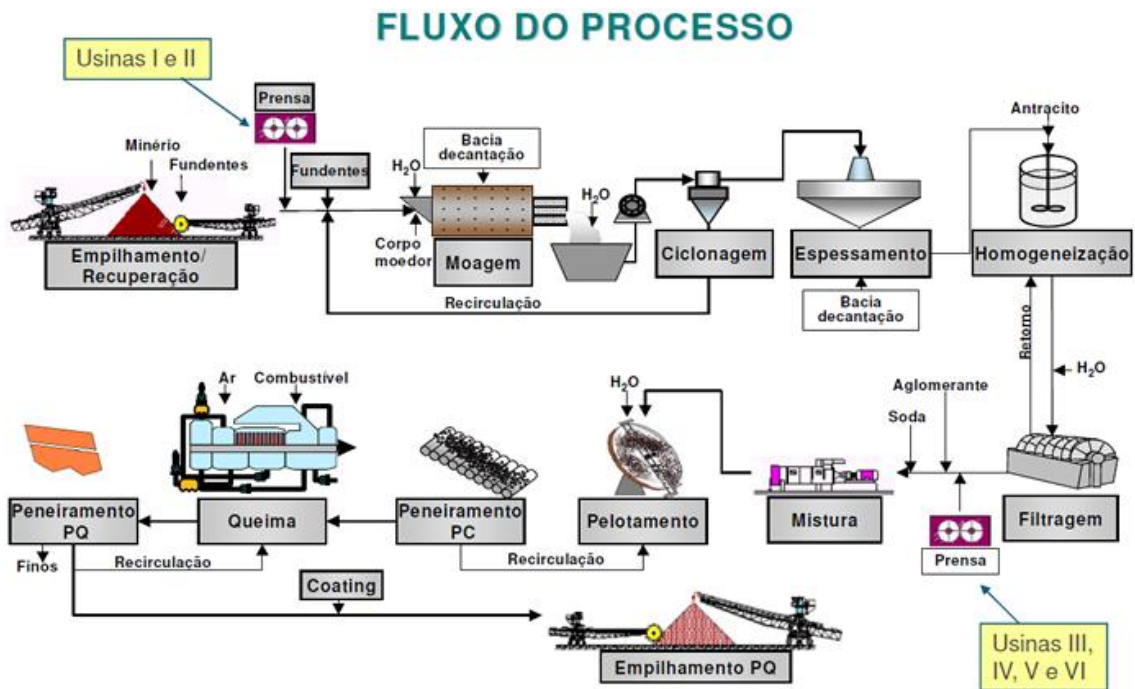
Figura 7 - Fluxo de Processo de Pelotização Usinas I a VI
