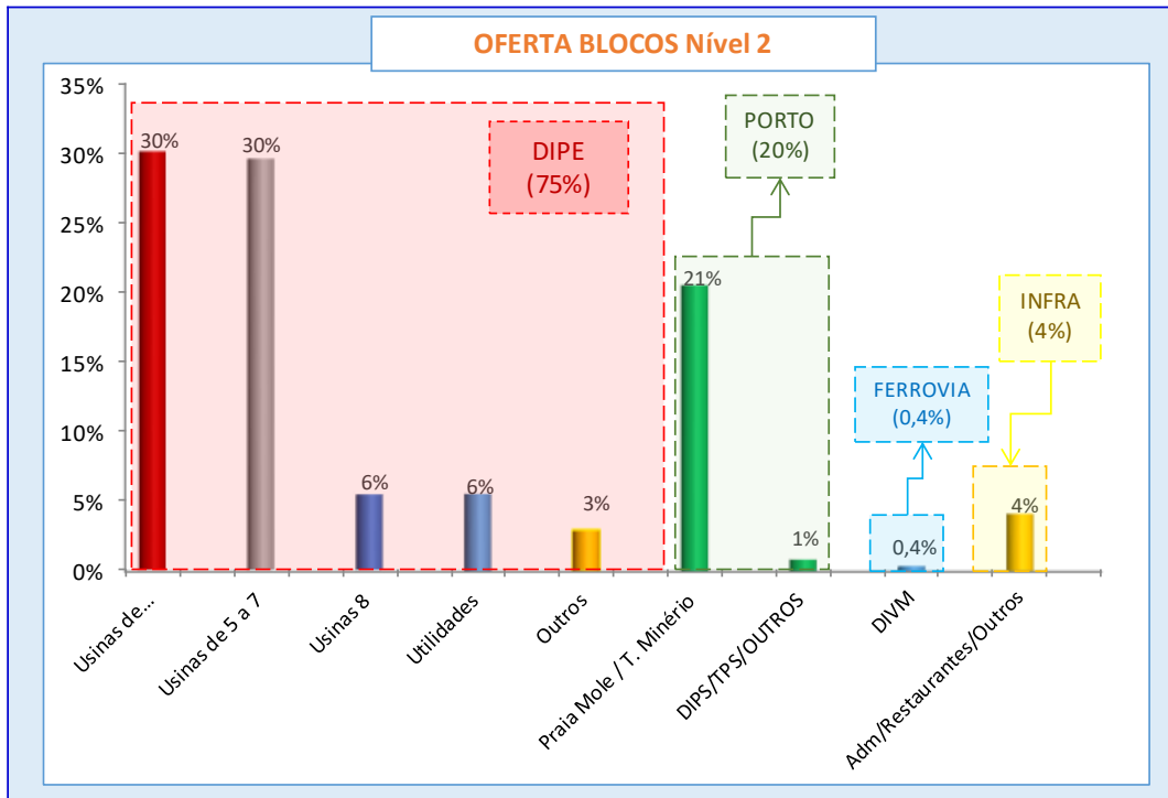
Figura 27 - Distribuição do consumo de água nova para os Blocos Consumidores
