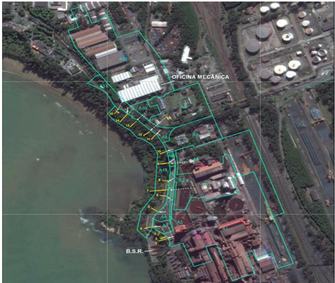
Figura 20 – Definição das áreas de contribuição do sistema de drenagem da região da DIPE
