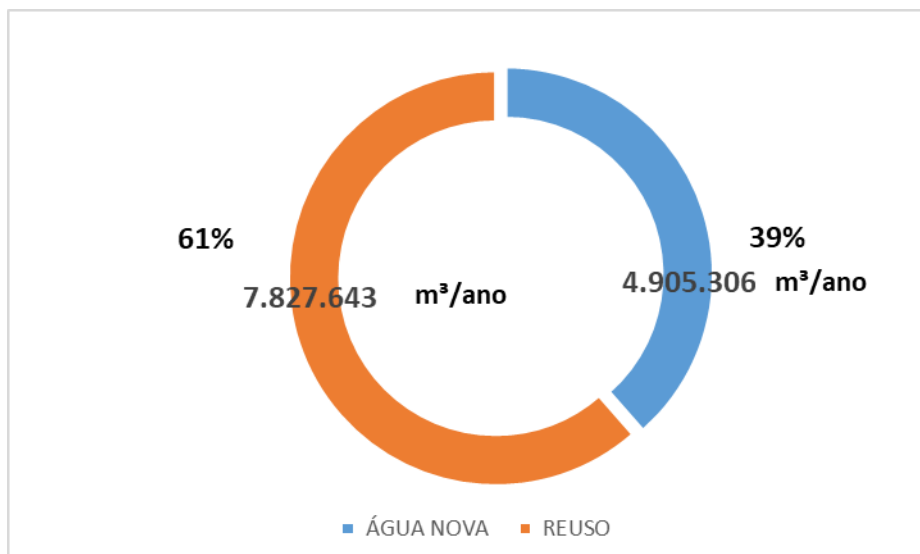
Figura 28 - Distribuição do percentual e da vazão média anual de toda água consumida na Unidade de Tubarão
