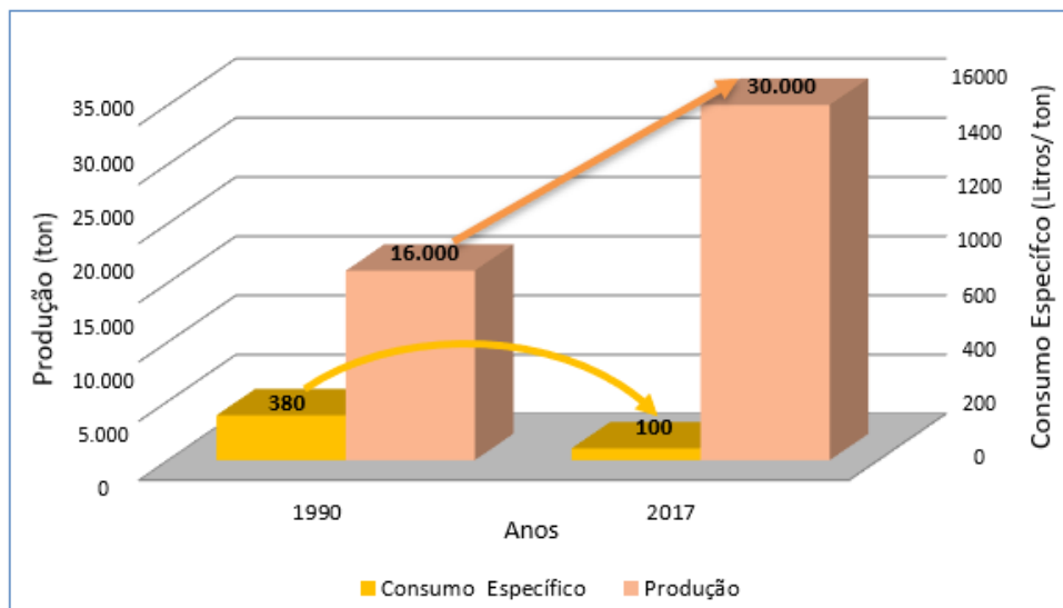
Figura 24 - Aumento da Produção x Redução do consumo específico de água
