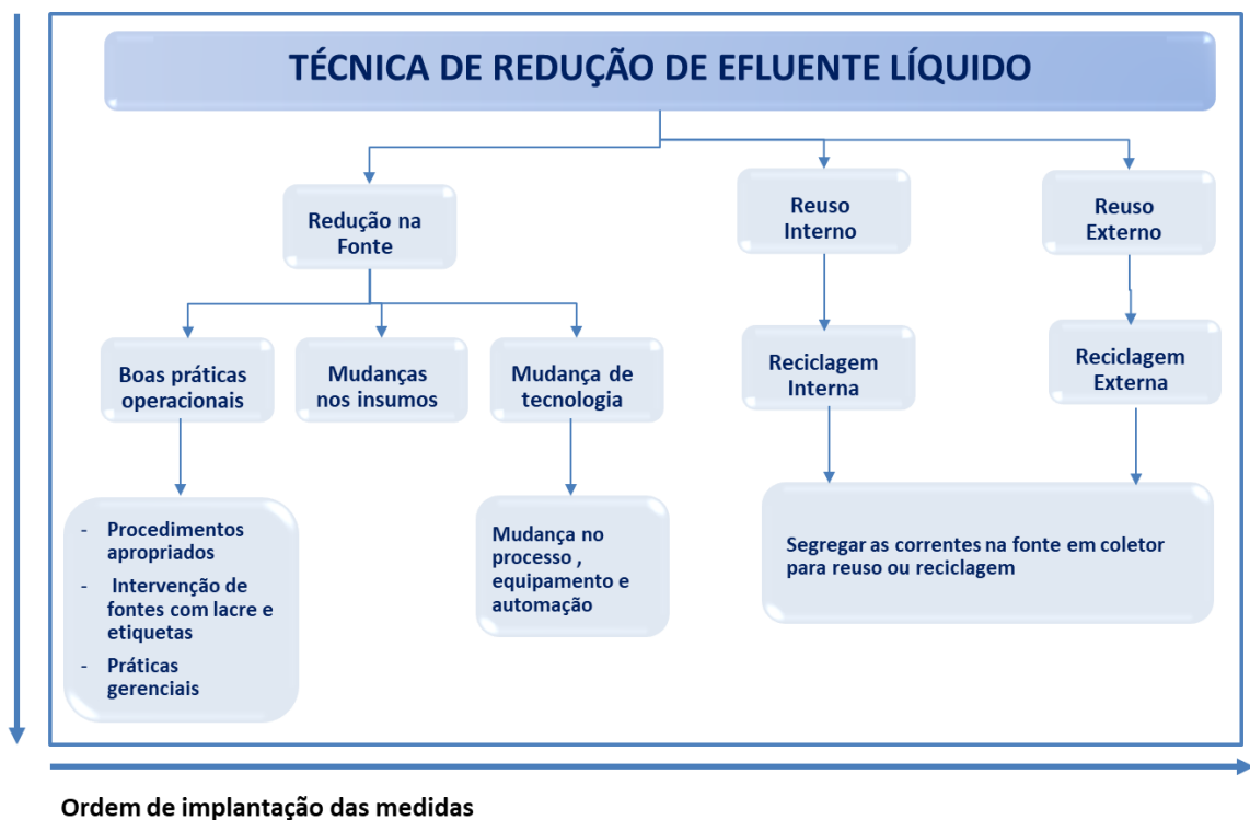
Figura 5 - Hierarquização de medidas técnicas preventivas para reduzir fontes de efluentes líquidos
