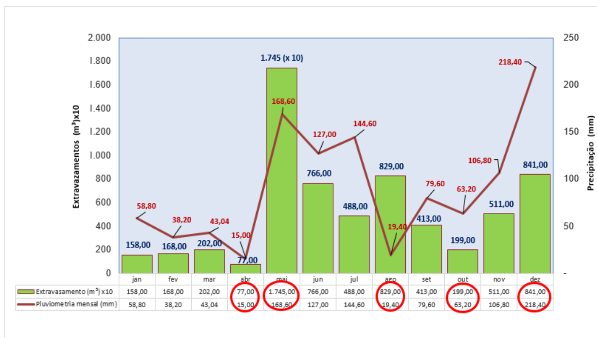
Figura 33 - Comparação dos Descartes (extravasamentos) ocorridos em Tubarão com a Precipitação mensal da região da DIPE no ano de 2017
