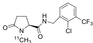
[ 11 C]GSK1482160
