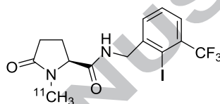
[ 11 C]I-GSK1482160
