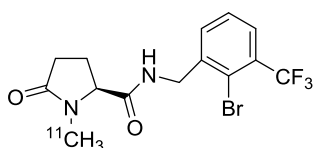
[ 11 C]Br-GSK1482160
