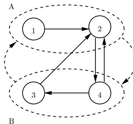
Abbildung 2.2: Ein Automat implementiert einen anderen Automaten (Virtualisierung).
