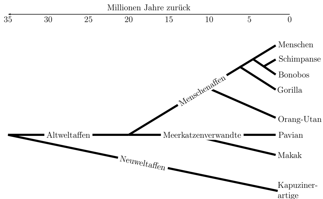
Abb. 8: Phylogenetischer Stammbaum ausgewählter Primaten. Basierend auf DNA-Vergleichen, modifiziert aus [314].
