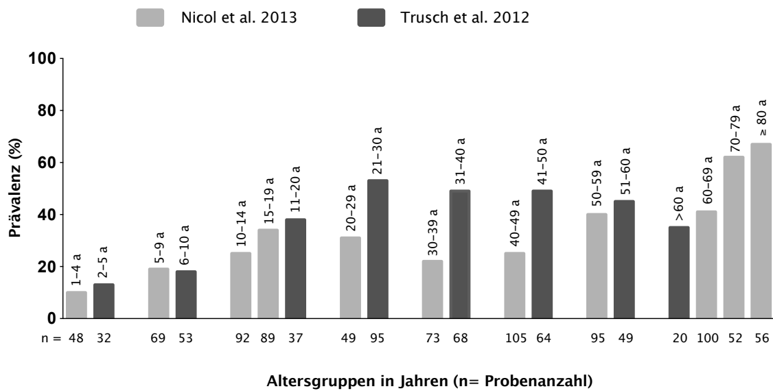
Abb. 17: Altersverteilung der Seroreaktivität gegen HPyV9. Bei gesunden Erwachsenen und Kindern in pädiatrischer Behandlung, [34, 176].
