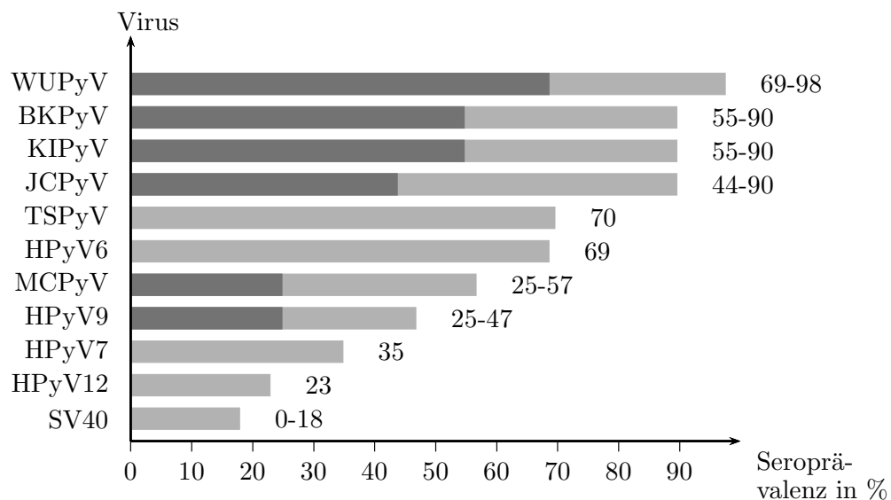
Abb. 7: Seroreaktivitäten gesunder Erwachsener gegen humane Polyomaviren und das Altweltaffen-Polyomavirus SV40. Existieren unterschiedliche Angaben zur Seroprävalenz sind jeweils der niedrigste (dunkelgrau) und der höchste (hellgrau) Wert dargestellt.
