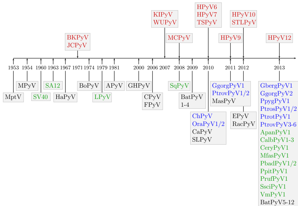
Abb. 2: Zeitachse der Entdeckungen der Polyomaviren. Humane Polyomaviren (rot), Menschenaffen-Polyomaviren (blau), andere Polyomaviren nicht-humaner Primaten (grün), andere Polyomaviren (schwarz).
