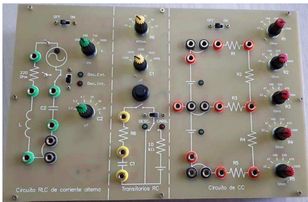
Figura 1. Placa autónoma PALC-1 en su versión actual.
