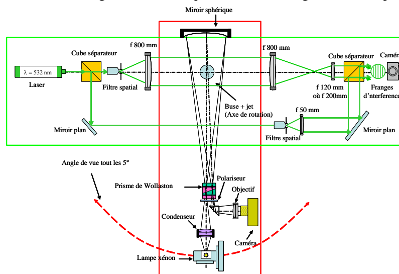
Figure 2 : Schéma du montage optique
