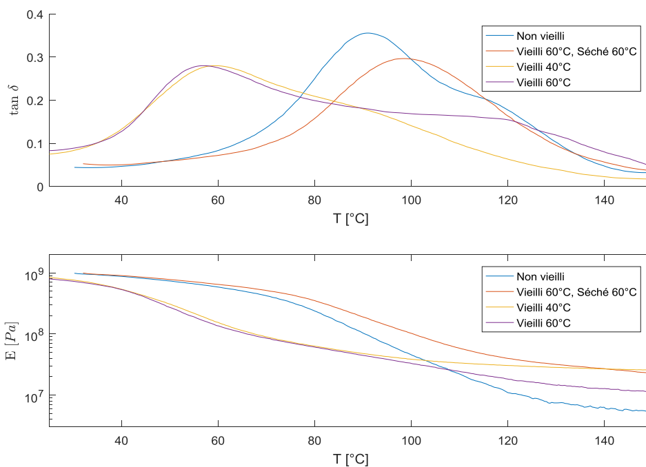
Figure 5: Essais DMA réalisés sur des échantillons ayant subi différents vieillissements (40 et 60°C)
