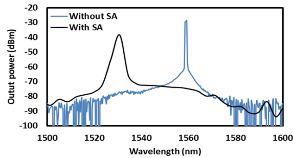
Figure 3. OSA trace without SA and with SA
