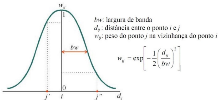
Figura 1: Função gaussiana. Fonte: Feitosa et al. , (2007, p. 69).
