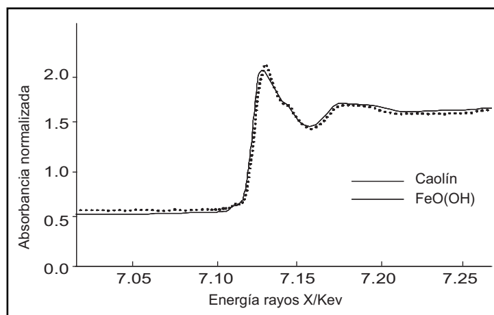
Figura 5. Espectro XANES del caolín superpuesto al espectro XANES del \text{FeO(OH)} .
