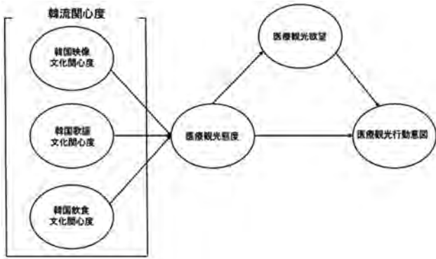
図3：研究モデル
