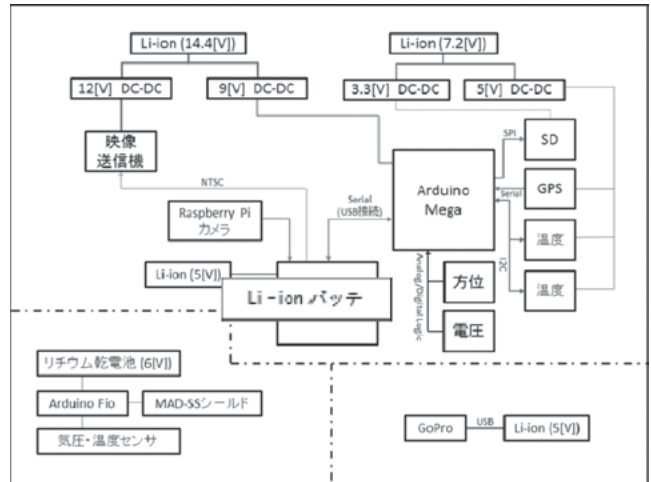
図9 ペイロード電装系ブロック図
