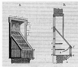
[居間の木製枠の植物置き場とその断面図]
