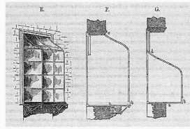
[居間の鉄枠の植物置き場とその断面図]
