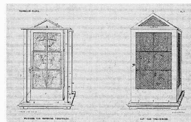
Wijziging van wardsche toestellen. Kap van traliewerk. ウォードの装置[ウォードの箱]の改造。格子作りの覆い
